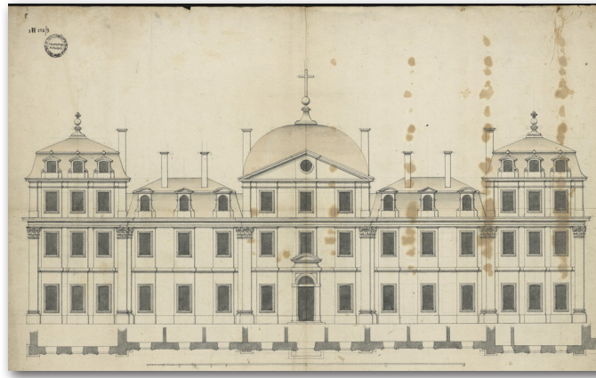
2. Projet anonyme de reconstruction de l'abbaye, façade nord regardant la rue Porte Guillaume. 1H/132/09/05.
