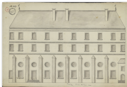
4. Élévation de la façade orientale du bâtiment de l'ancien dortoir surmonté de deux niveaux de cellules. Projet anonyme, c. 1652. 1H/132/09/02.
